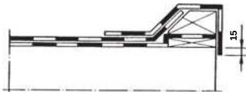
Bild 1. Saneringsarbete, takskägg med upphöjd kant, enkelt tätskikt.
