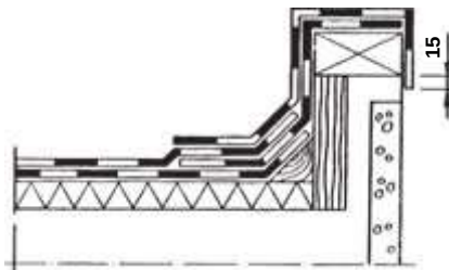
Bild 5. Talskäg, dubbelt
