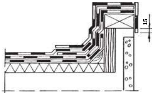
Bild 6. Takskägg, tredubbelt täktskikt.
