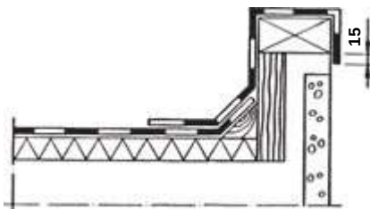
Bild 4. Talskäg, enkelt tätskikt.
