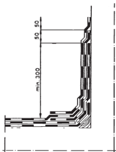
Bild 9. Upp mot vägg, tredubbel tätskikt.
