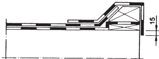
Bild 1. Saneringsarbete, takskägg med upphöjd kant, enkelt tät-skikt.
