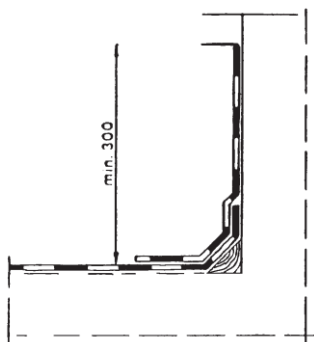
Bild 7. Upp mot vägg, enkelt täktskikt.
