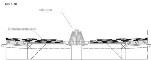
Bild 10. Takbrunn. Brunnen ska ligga minst 20 mm lägre än den övriga takytan.
