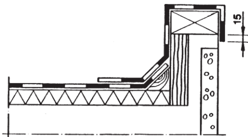
Bild 4. Takskägg, enkelt tätskikt.
