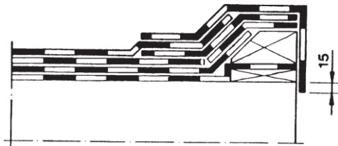
Bild 3. Saneringsarbete, upphöjd kant, tredubbelt tätskikt.
