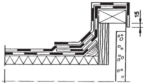
Bild 5. Takskägg, dubbelt tätskikt.
