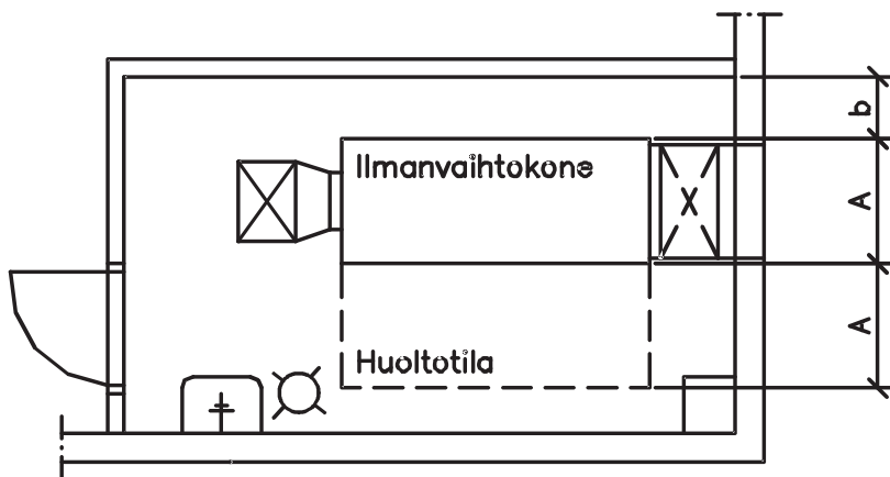
Kuva 4. Koteloidun ilmanvaihtokoneen huoltotilan sijoitus ja mitoitus esimerkki. A on ilmanvaihtokoneen leveys ja b on 0,4 kertaa ilmanvaihtokoneen korkeus tai vähintään 400 mm.
